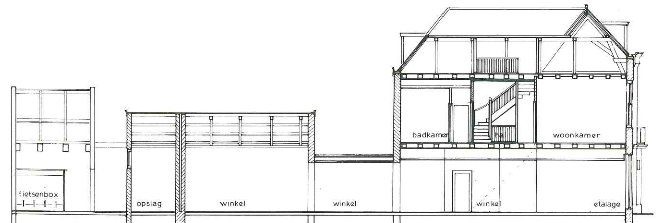
19. Twee doorsneden van het pand, na de verbouwing van 1985.
