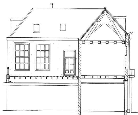
20. Vooraanzicht (boven) en zijgevel + doorsnede (onder), na de verbouwing van 1985.
