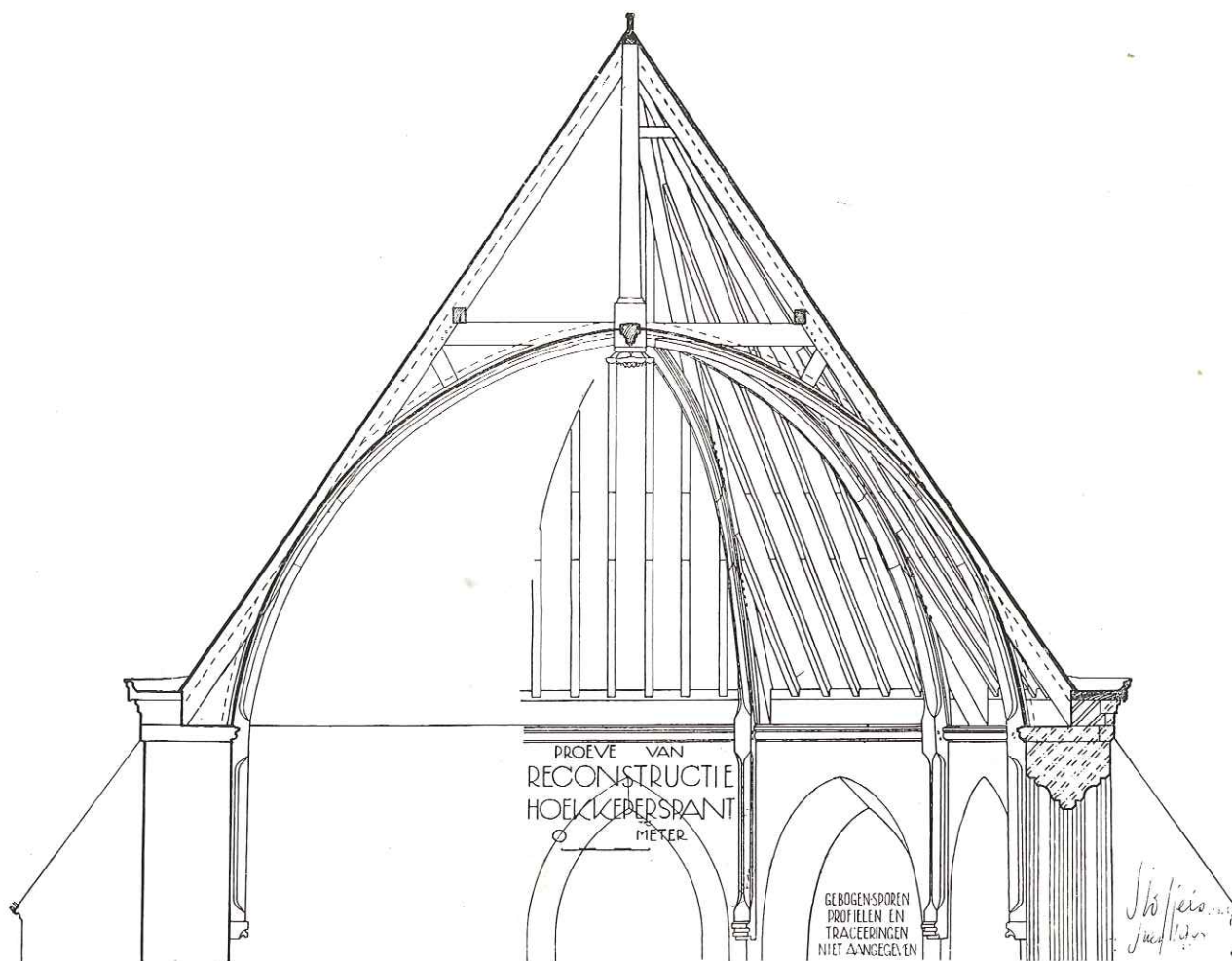
2. Reconstructie van de kap der Kloosterkerk.
