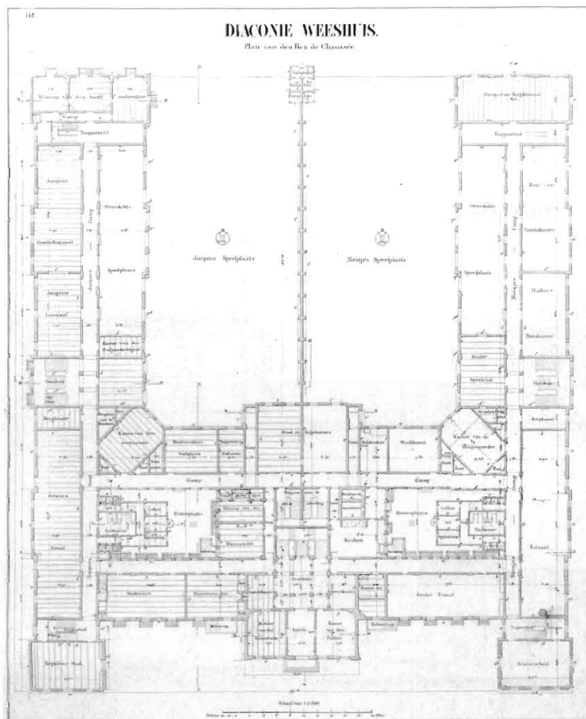
Plattegrond begane grond Diaconie weeshuis, E. Saraber. (GA)
