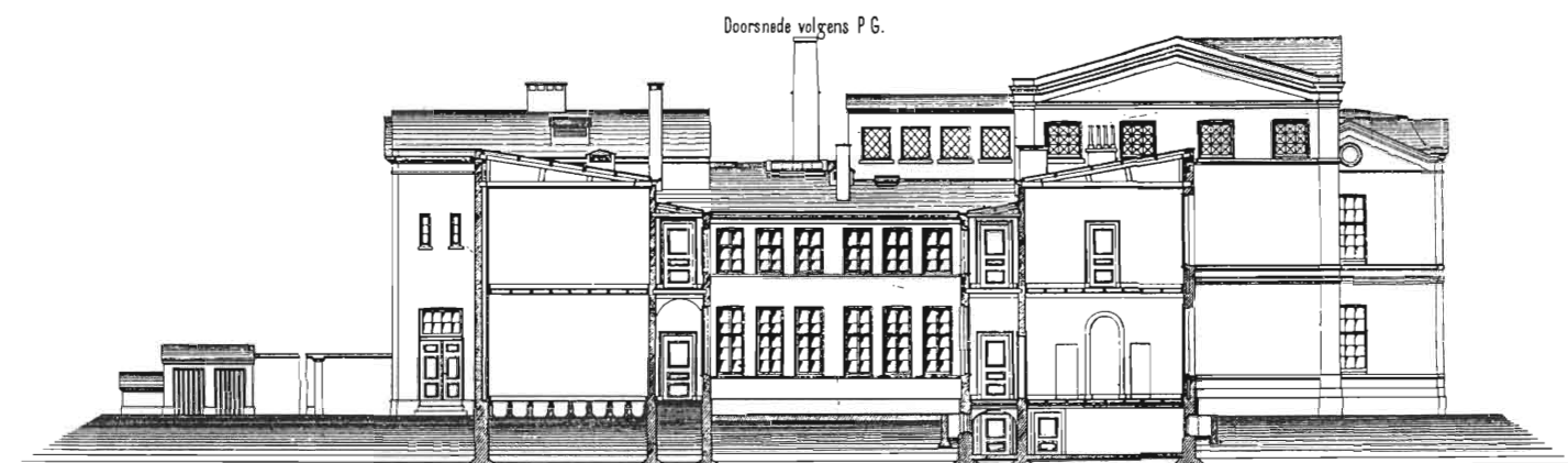
Doorsnede hoofdpaviljoen en deel zijvleugel en doorsnede verbindingsstuk tussen hoofd- paviljoen en hoekpaviljoen, E. Saraber. (GA, bnr. 133, inv.nr. 1758)
