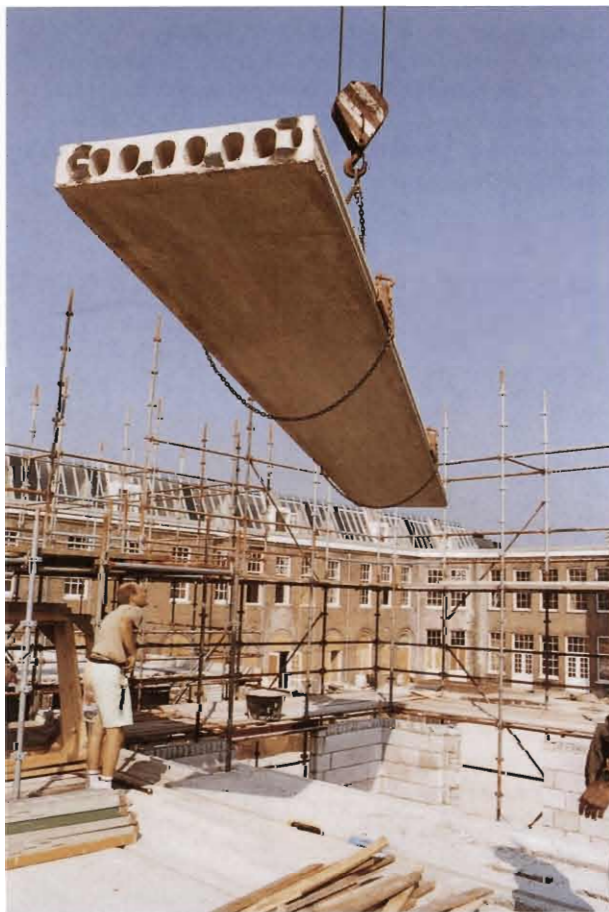
Het aanbrengen van de verdiepingsvloer in het poortgebouw.
