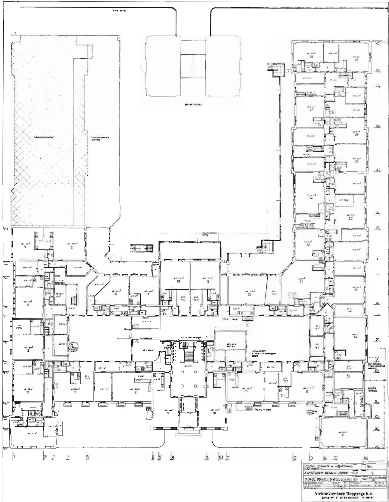
Plattegrond van de begane- grond na de restauratie.
