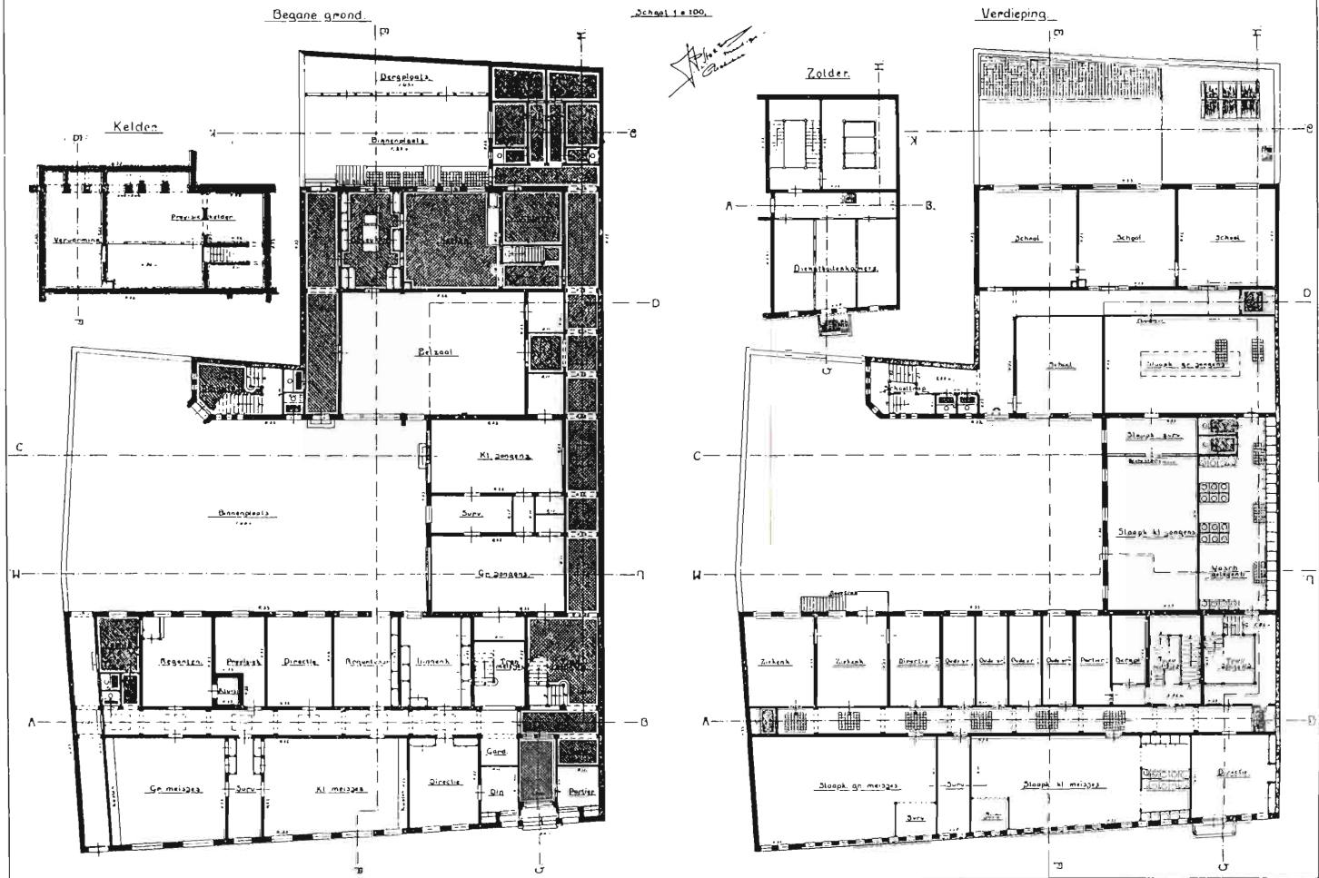
Plattegronden van de nieuwbouw van het Waalse weeshuis uit 1901. (GA, bnr.241, inv.nr.1462)
