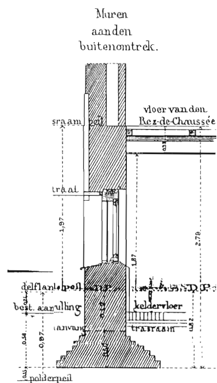
Detail van de fundering zoals op de oorspronkelijke tekenin- gen staat aangegeven. (GA).
